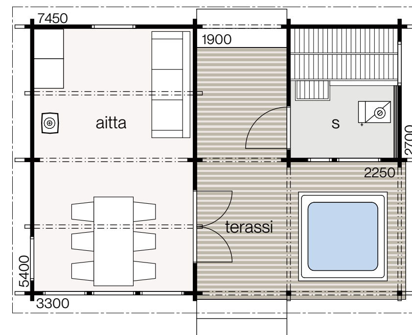
LEHTO 25A | KOKONAISKÄYTTÖALA 41,0 m 2 | KERROSALA 25,0 m 2
