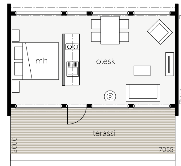
GLASS HOUSE 30A | KOKONAISKÄYTTÖALA 44 m 2 | KERROSALA 30 m 2
