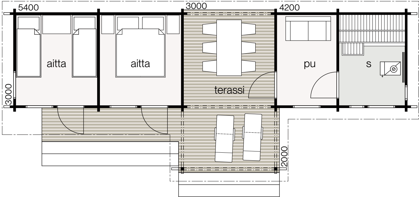
LUOTO 30A | KOKONAISKÄYTTÖALA 51,0 m 2 | KERROSALA 30,0 m 2
