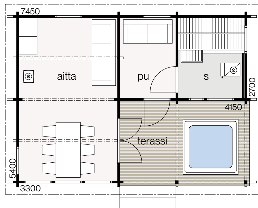
LEHTO 30A | KOKONAISKÄYTTÖALA 42,0 m 2 | KERROSALA 30,0 m 2
