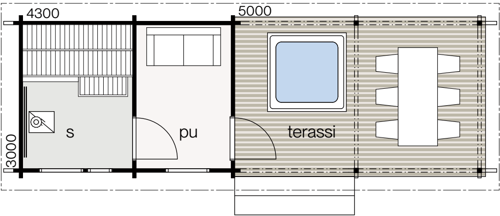
LUOTO 14A | KOKONAISKÄYTTÖALA 30,0 m 2 | KERROSALA 13,5 m 2
