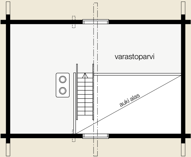
Kuusela 25 1-krs, asiakkaan muunnosmalli
