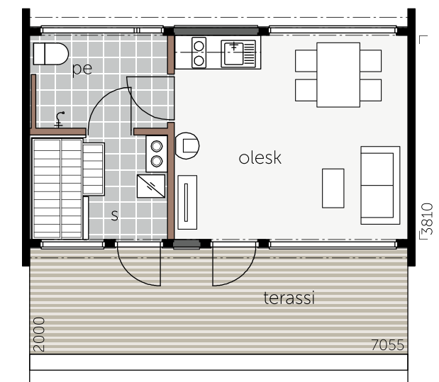
GLASS HOUSE 30B | KOKONAISKÄYTTÖALA 44 m 2 | KERROSALA 30 m 2
