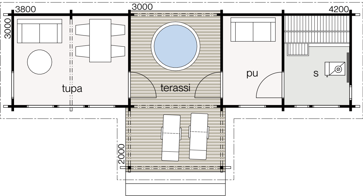
LUOTO 25A | KOKONAISKÄYTTÖALA 41,0 m 2 | KERROSALA 25,0 m 2
