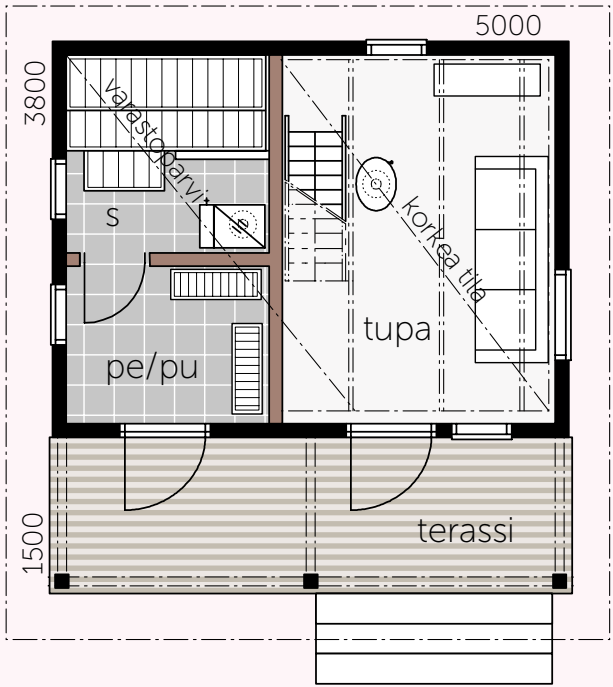
NALLE 20C KERROSALA KOKONAISKÄYTTÖALA 1-KERROKSISENA: KOKONAISKÄYTTÖALA PARVELLA: 20 m 2 28 m 2 35,5 m 2
