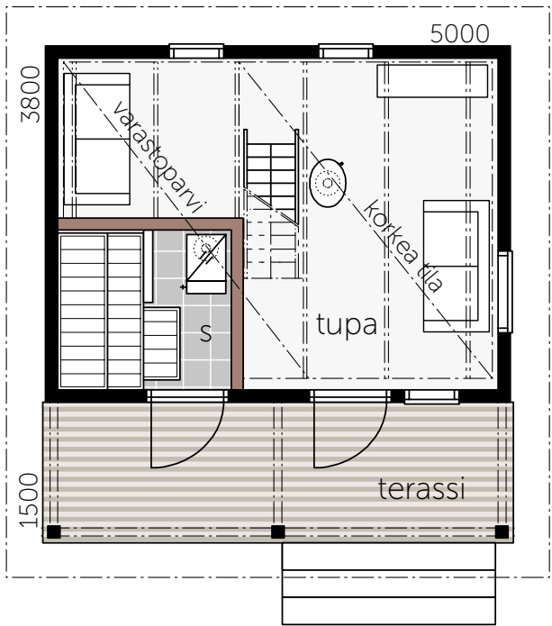
NALLE 20B KERROSALA KOKONAISKÄYTTÖALA 1-KERROKSISENA: KOKONAISKÄYTTÖALA PARVELLA: 20 m 2 28 m 2 35,5 m 2
