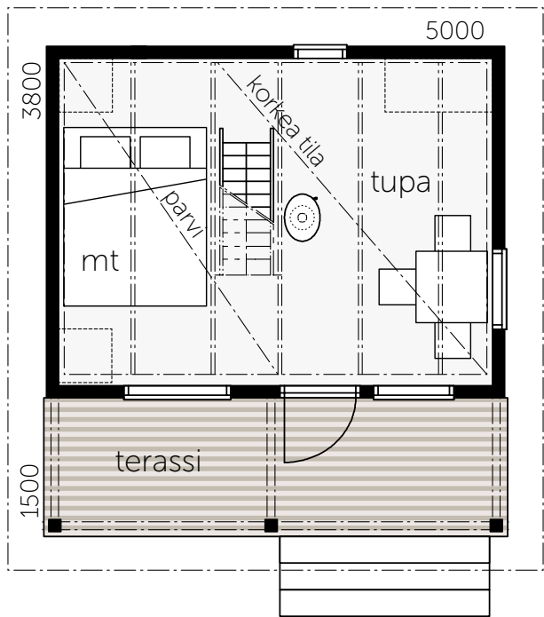
NALLE 20A KERROSALA KOKONAISKÄYTTÖALA 1-KERROKSISENA: KOKONAISKÄYTTÖALA PARVELLA: 20 m 2 28 m 2 34,5 m 2
